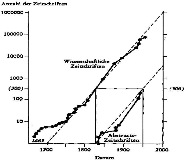
Abbildung 1: Gesamtzahl der Gründungen von wissenschaftlichen Zeitschriften und Abstract-Zeitschriften als einer Funktion der Zeit. Man beachte, dass die Ausgleichsgerade die 1700 beginnt, eindeutig zu steil eingezeichnet wurde, um die Verdopplungsrate mit 15 Jahren zu dramatisieren
